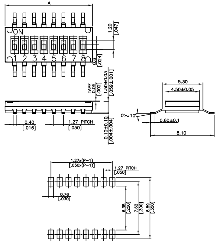
P.C.B. LAYOUT
