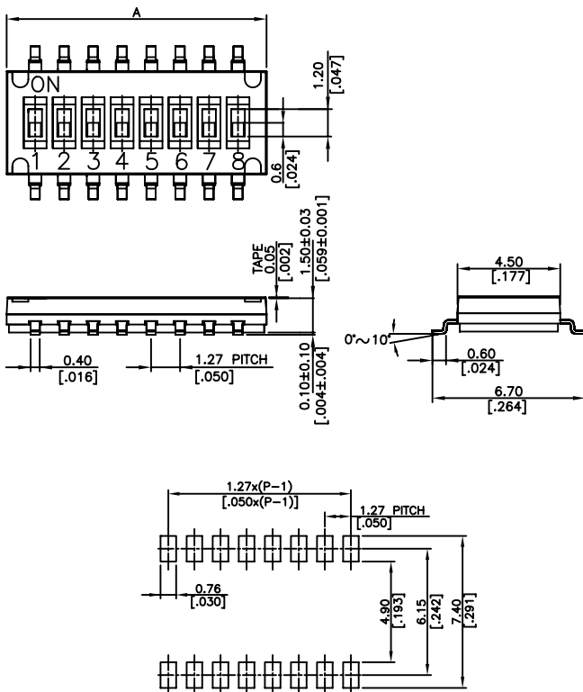
P.C.B. LAYOUT
